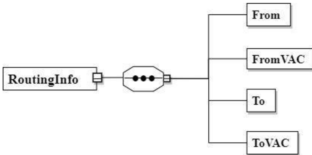
圖 27-3、SummaryResult /RoutingInfo 訊息結構圖
